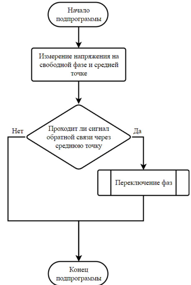
Измерение обратной ЭДС
